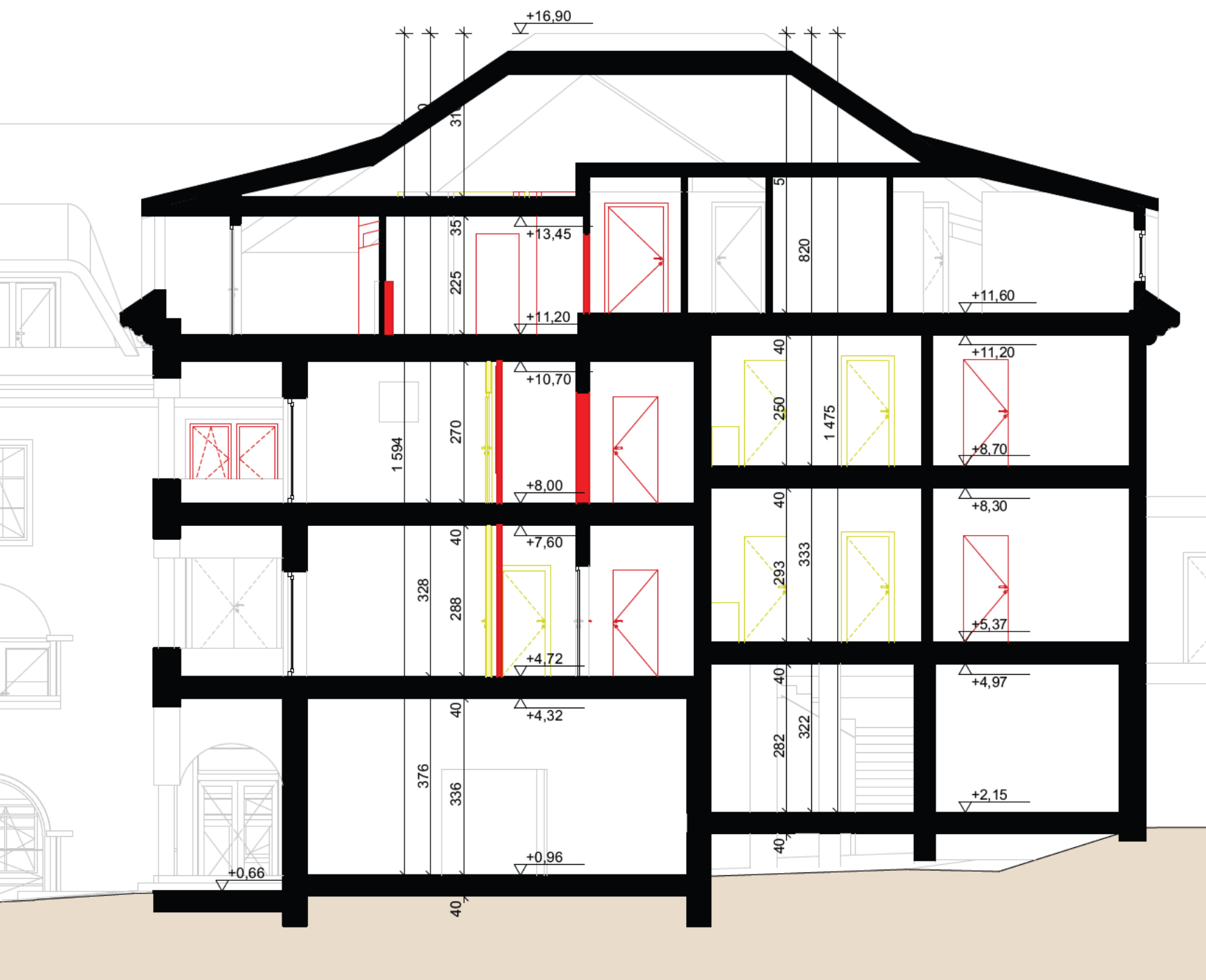
Schnitt B-B
